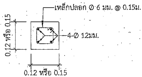
รูปตัด A-A
