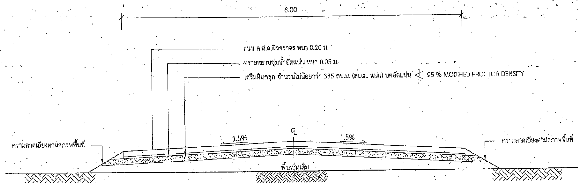
รูปตัด A NOT TO SCALE
