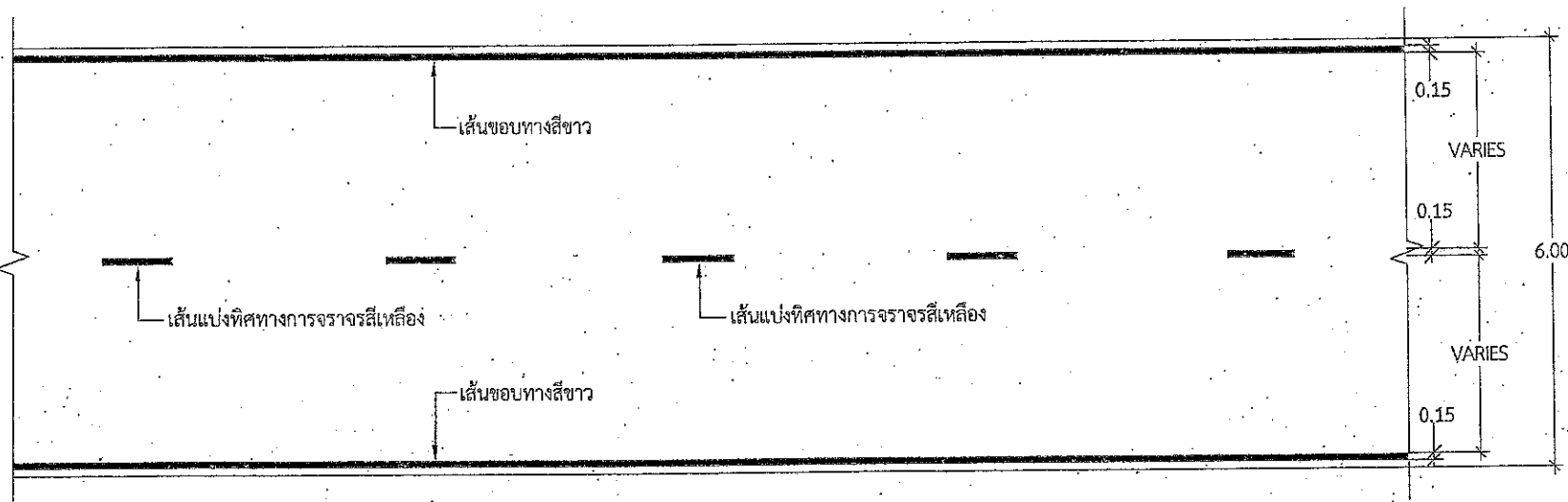
มาตรฐานการตีเส้นขอบทางสีขาว (มิติเป็นเมตร)
