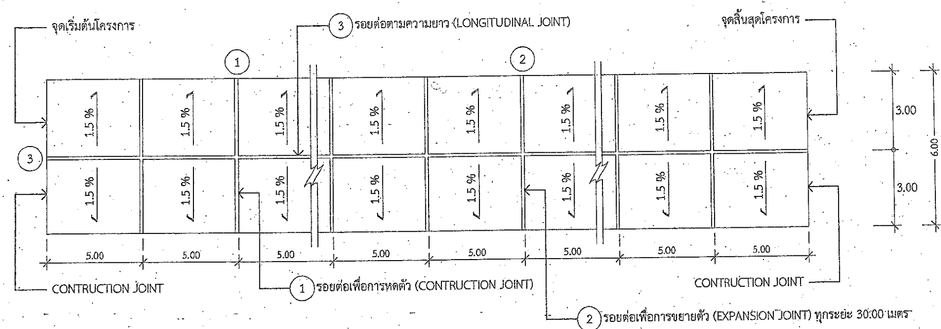
แปลนพื้นถนน ค.ส.ล. NOT TO SCALE
