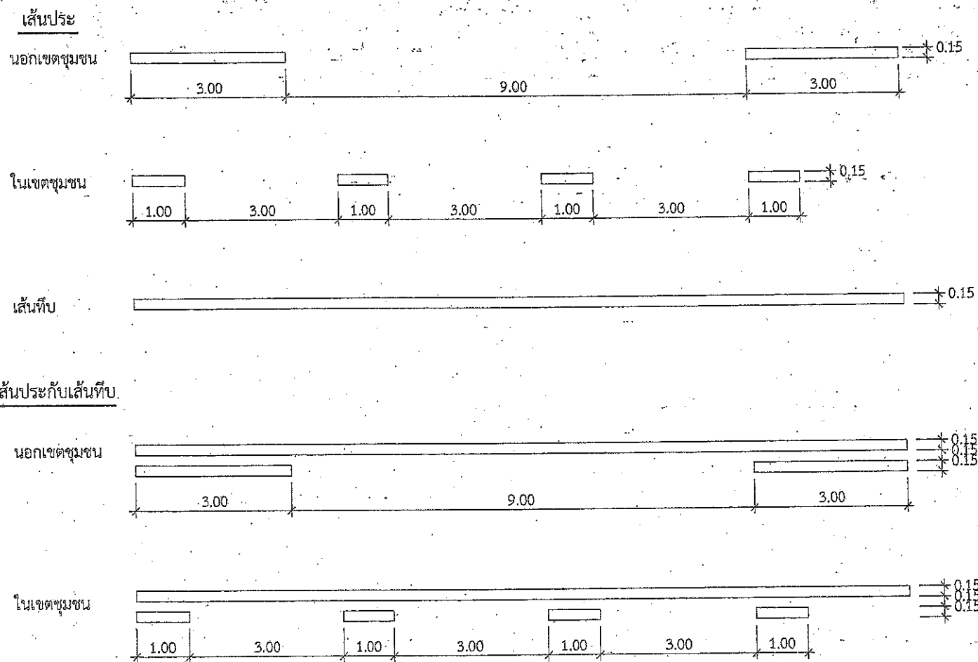
มาตรฐานเส้นแบ่งช่องจราจรสี่เหลี่ยม (มิติเป็นเมตร)
