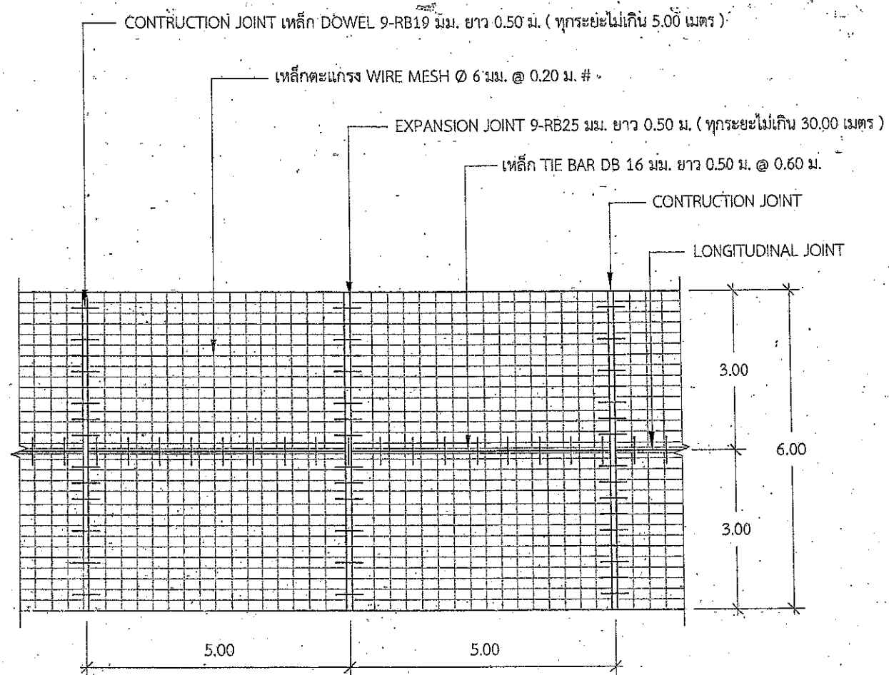
แปลนการวางตะแกรงเหล็ก
